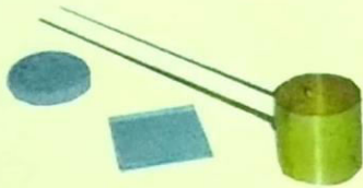
Le-Chatlier Mould
