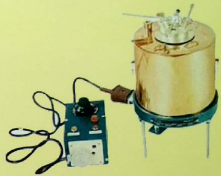
Abel Flash Point Apparatus
